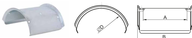
Auflage aus Stahl mit zwei Flanschen
