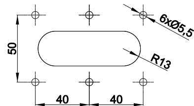
Rozmieszczenie otworów montażowych Mounting holes location Die Lage der Montagebohrungen
