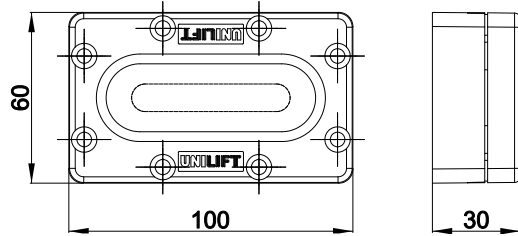
Rozmieszczenie otworów montażowych Mounting holes location Die Lage der Montagebohrungen
